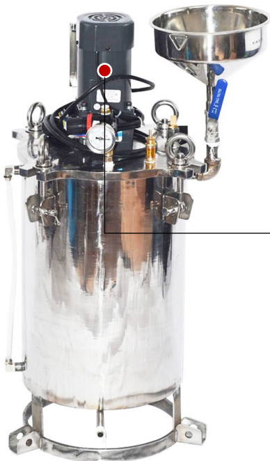
Agitator Tank
